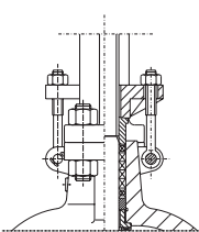
Скоба для DN 150 и выше
